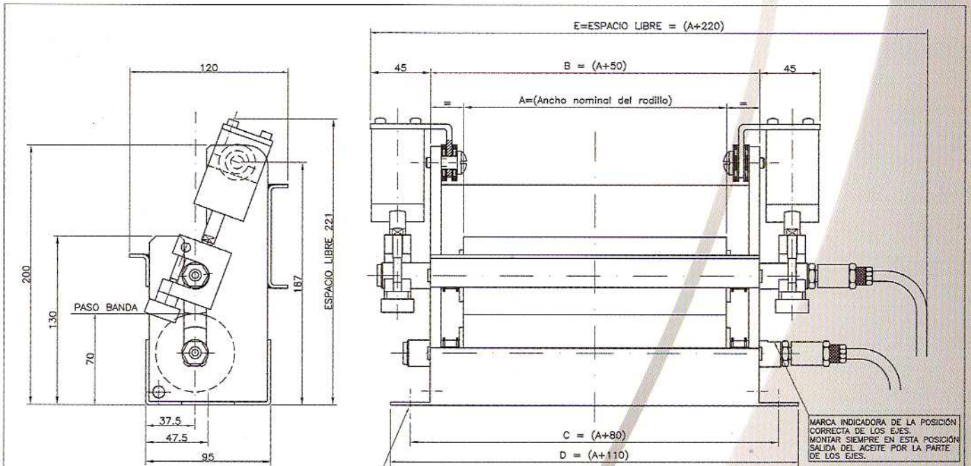
FIJACION CON DOS TORNILLOS M8
