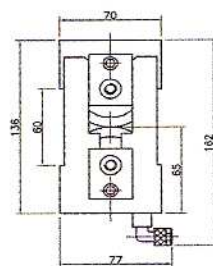
DIMENSIONES RODILLO SIN BASTIDOR
