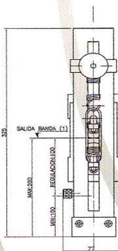
(1)—AJUSTAR A LA ALTURA DE TRABAJO DE LA MATRIZ
