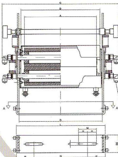
SEZ. A-A'
